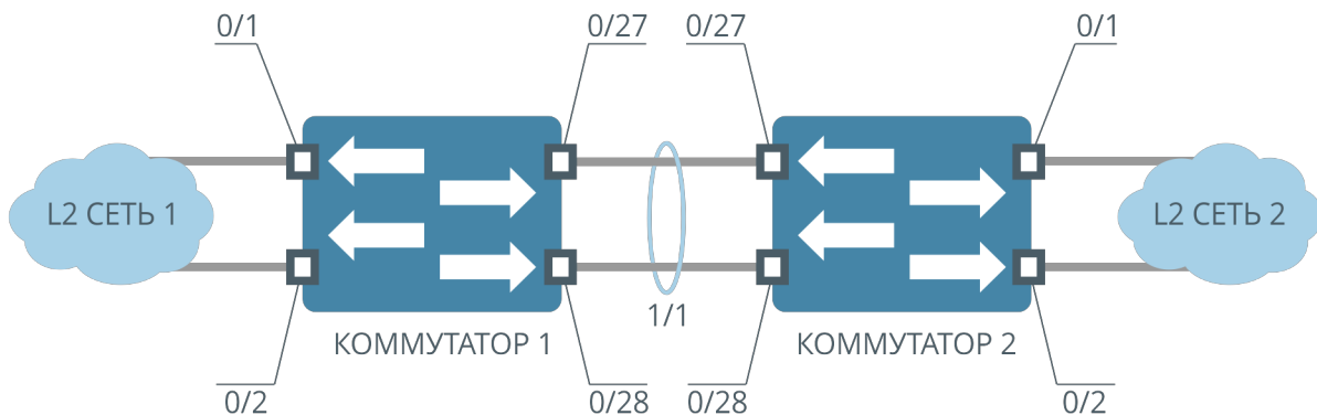
Рисунок 14. Пример агрегации каналов для двух L2-сетей
