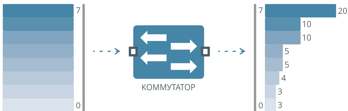
Рисунок 65. Алгоритм Weighted Round Robin
