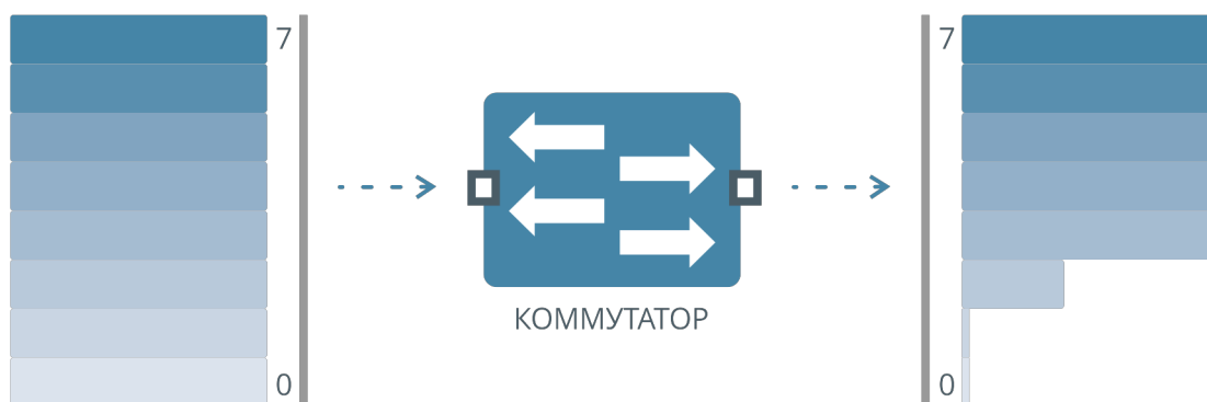
Рисунок 64. Алгоритм Strict Priority
