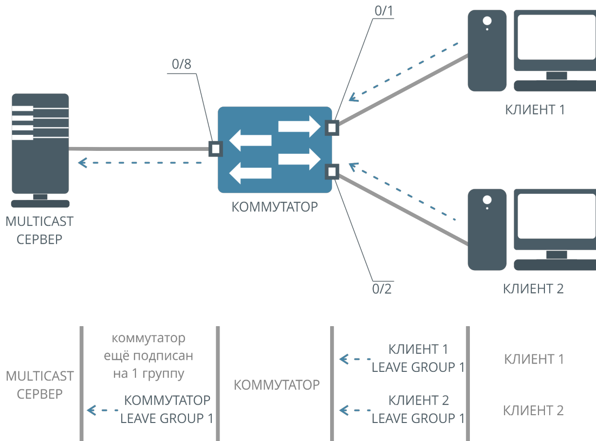
Рисунок 51. Режим IGMP Proxy Reporting, Leave
