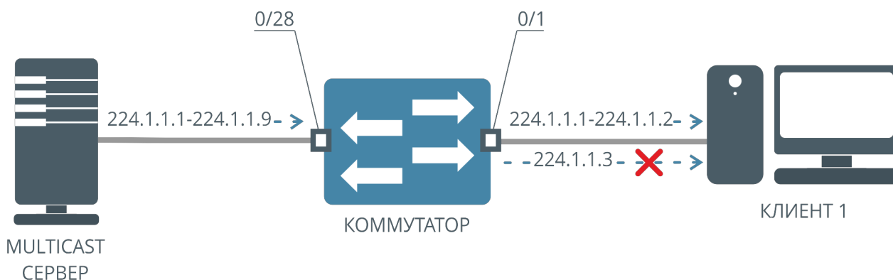
Рисунок 43. Схема работы ограничения количества multicast-групп на клиентском интерфейсе
