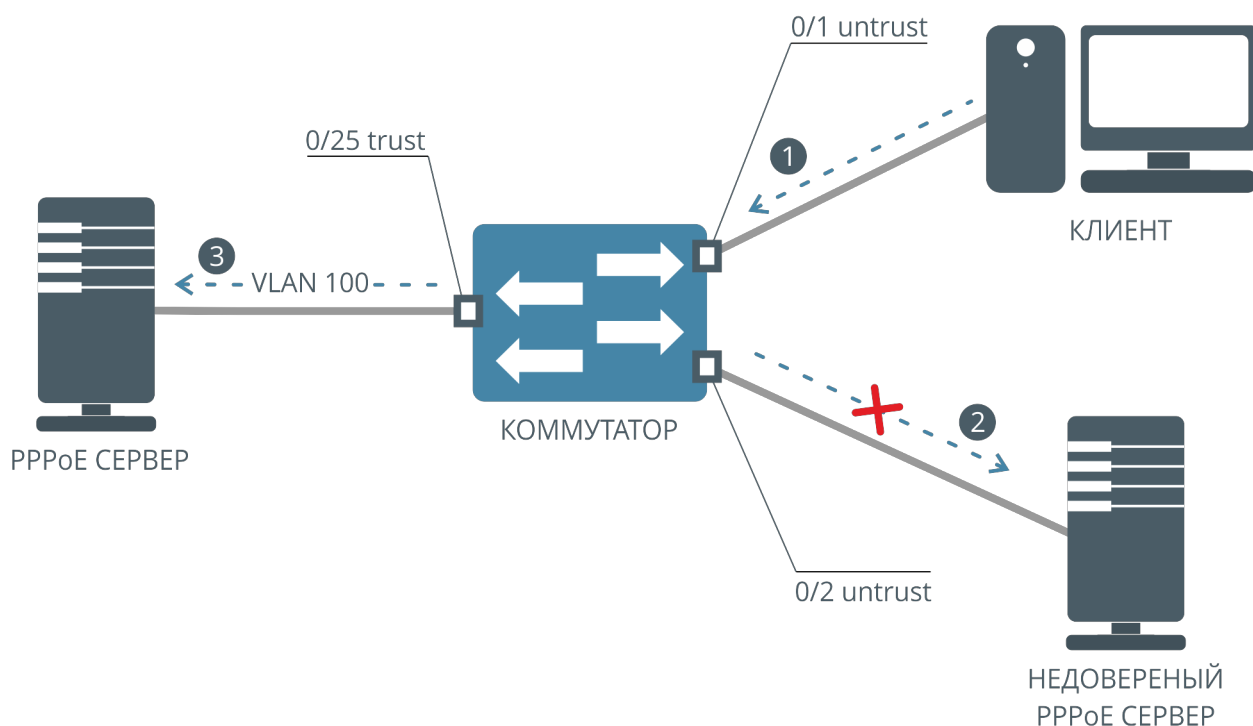
Рисунок 53. Схема работы PPPoE Snooping
