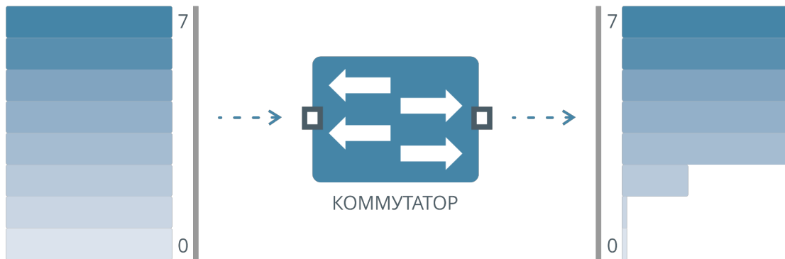
Рисунок 64. Алгоритм Strict Priority
