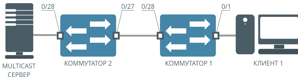
Рисунок 45. Схема работы IGMP Proxy
