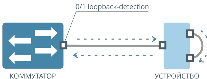
Рисунок 16. Схема работы службы обнаружения петель
