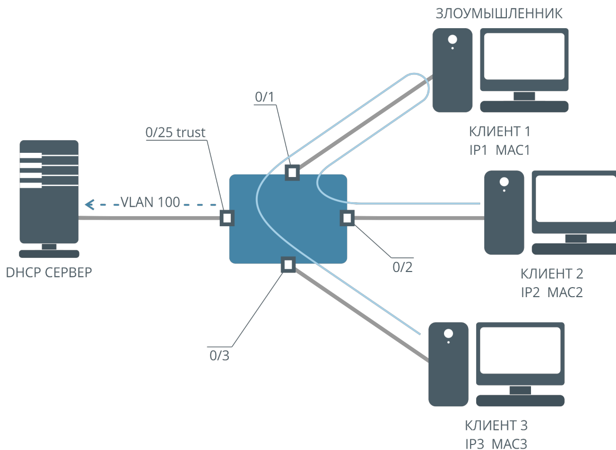
Рисунок 59. Упрощенная схема атаки с подменой MAC-адресов
