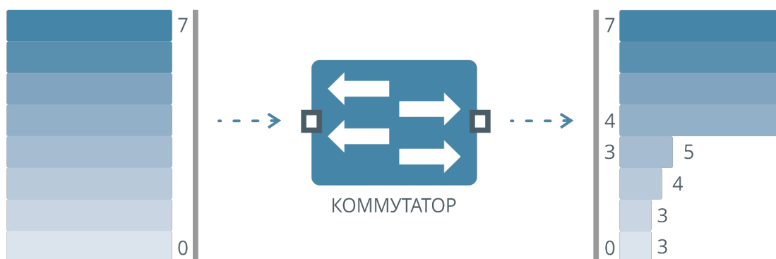
Рисунок 66. Алгоритмы Strict Priority и Weighted Round Robin одновременно
