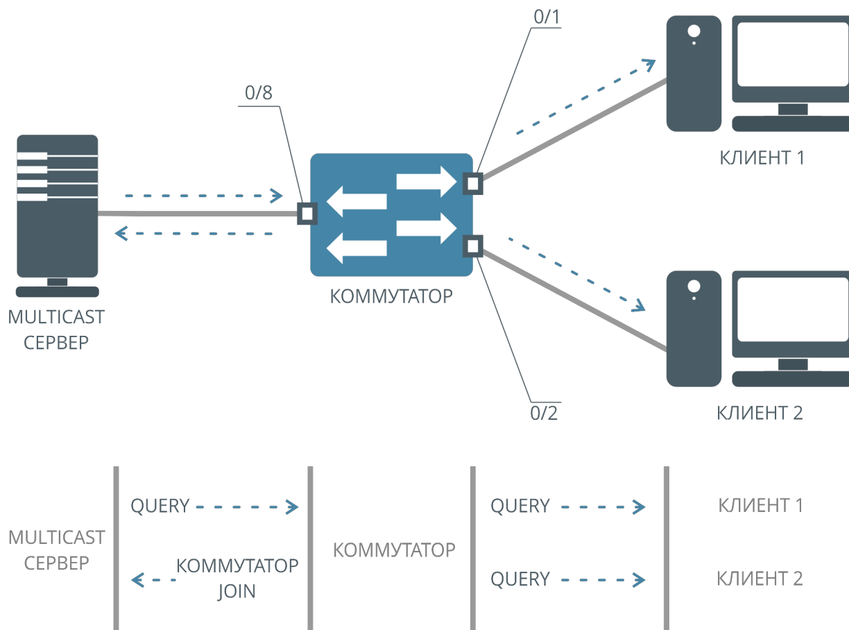
Рисунок 52. Режим IGMP Proxy Reporting, Query
