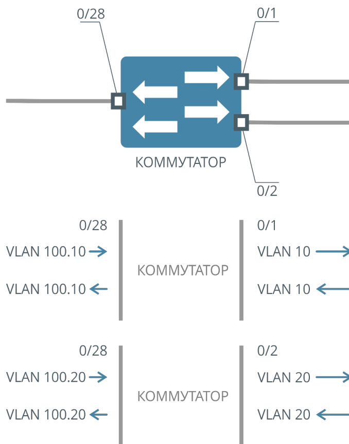
Рисунок 31. Схема прохождения клиентских пакетов
