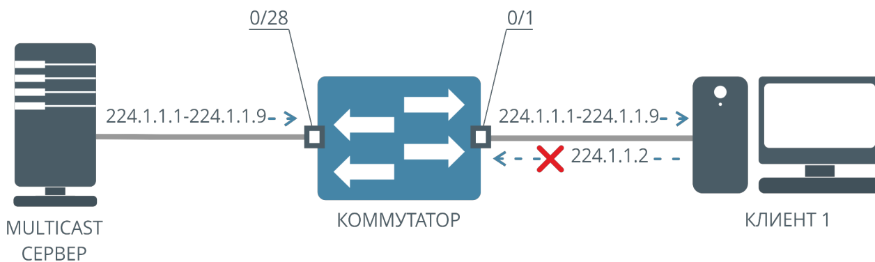
Рисунок 44. Схема работы статических групп
