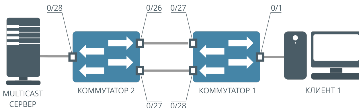
Рисунок 41. Схема работы IGMP dynamic mrouter
