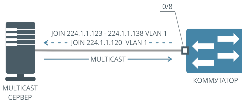
Рисунок 49. Схема работы автоматической подписки на группы
