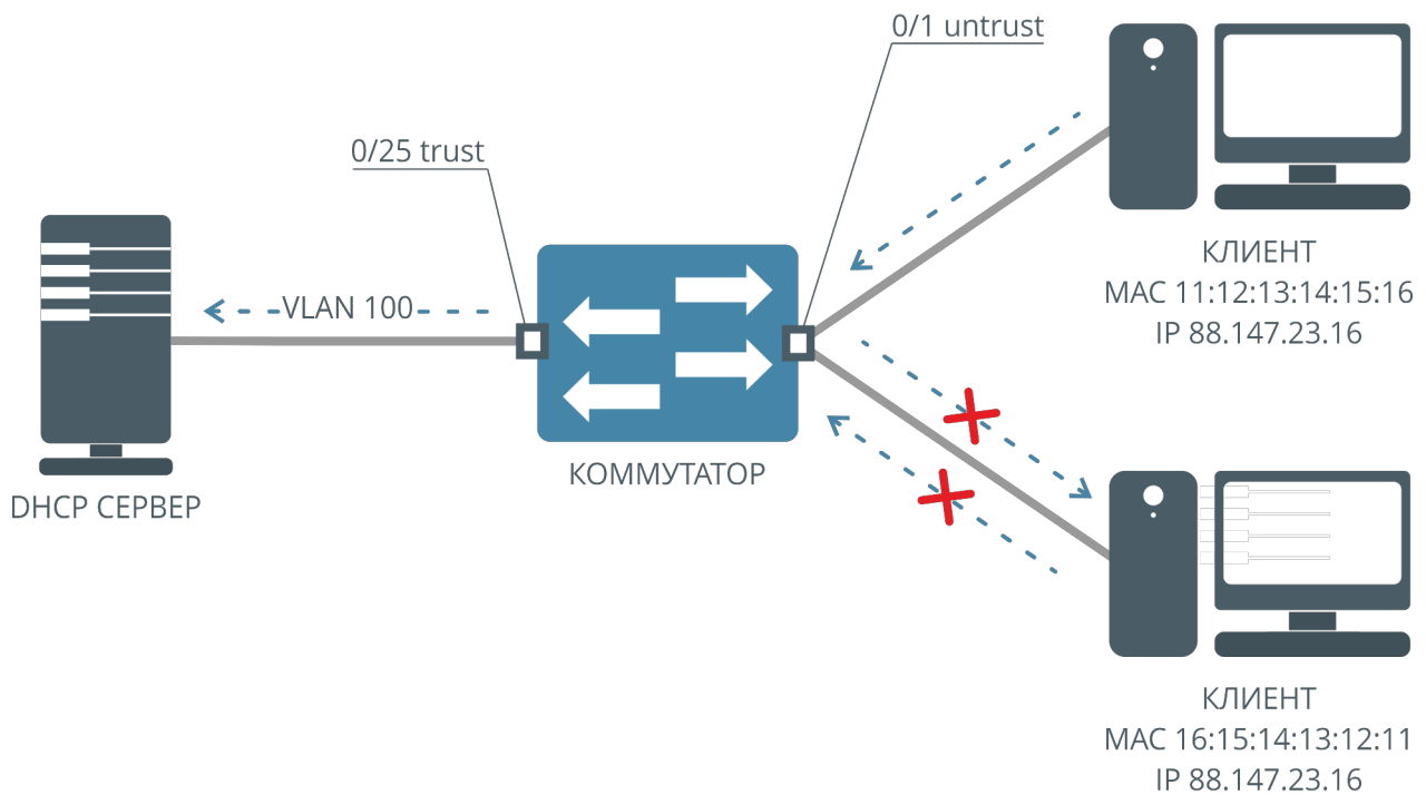
Рисунок 58. Схема работы DHCP IP Source Guard
