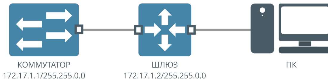
Рисунок 4. Подключение ПК к коммутатору через шлюз
