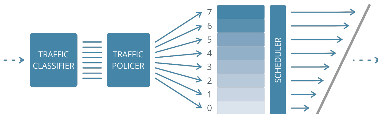
Рисунок 63. Механизм работы QoS на коммутаторах АЛСиТЕК
