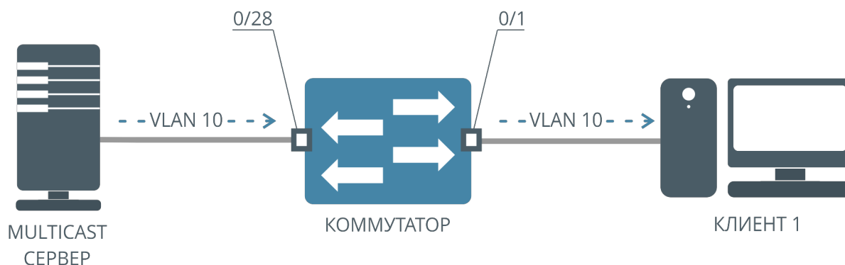
Рисунок 47. Схема работы IGMP Querier
