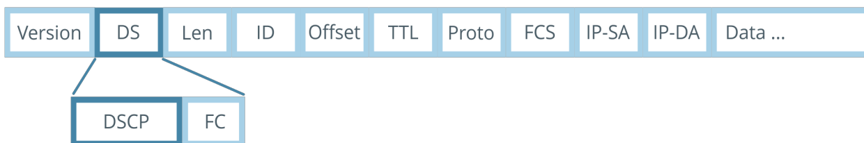
Рисунок 62. Положение метки DSCP в заголовке IP-пакета
