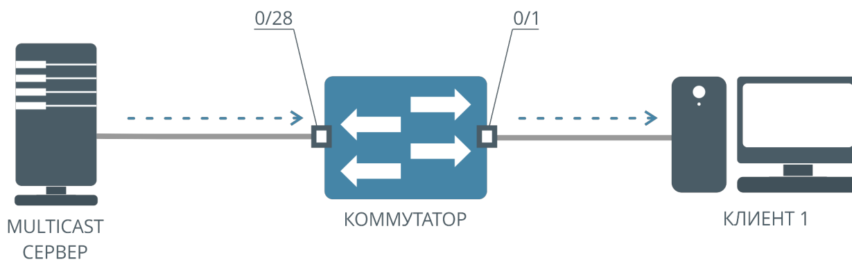
Рисунок 46. Схема подключения с одним клиентом
