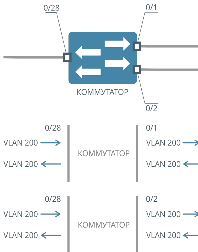
Рисунок 32. Схема прохождения трафика IPTV
