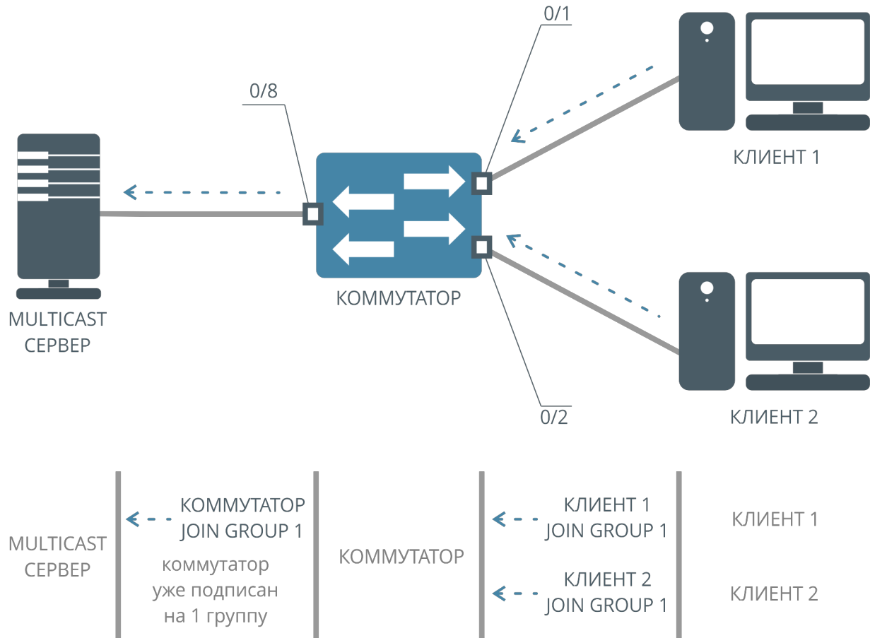
Рисунок 50. Режим IGMP Proxy Reporting, Join
