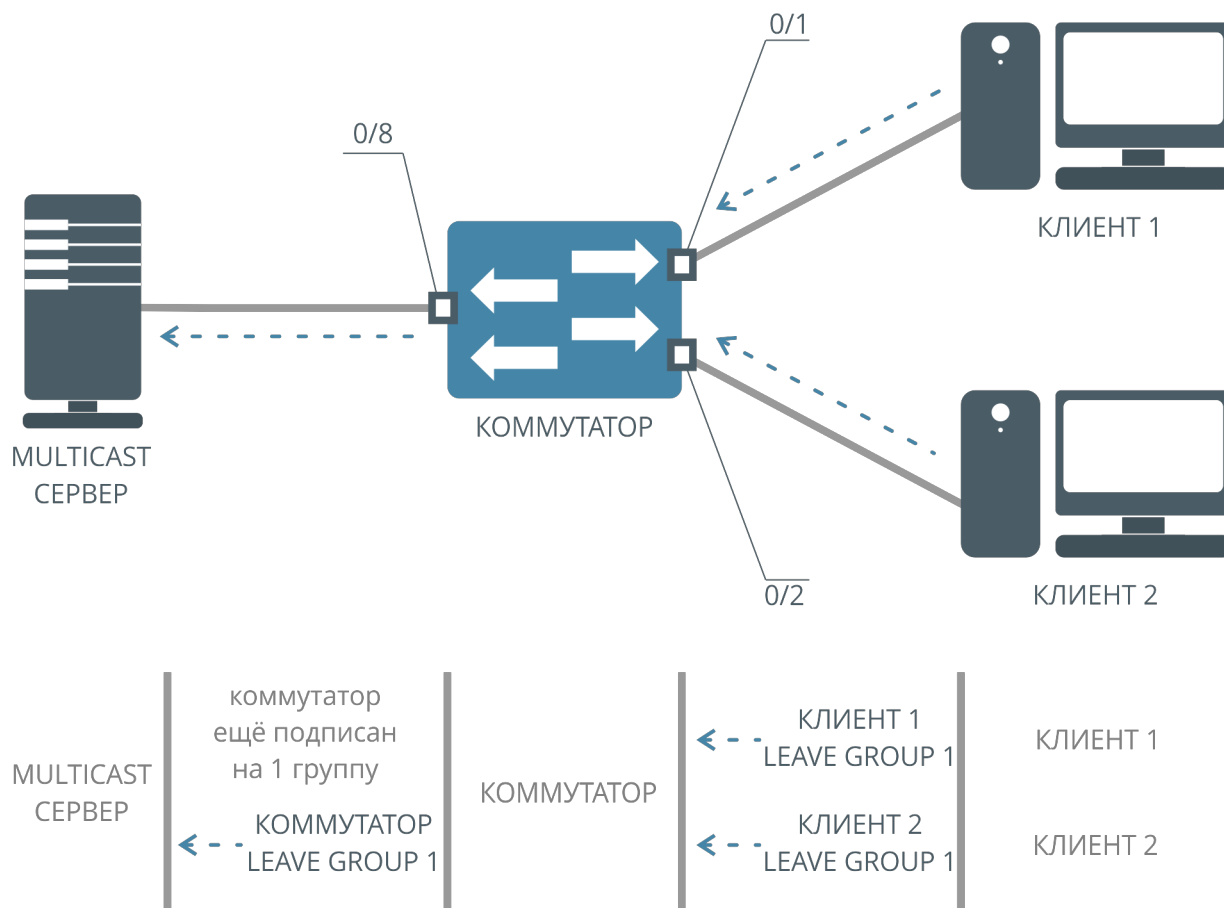
Рисунок 51. Режим IGMP Proxy Reporting, Leave
