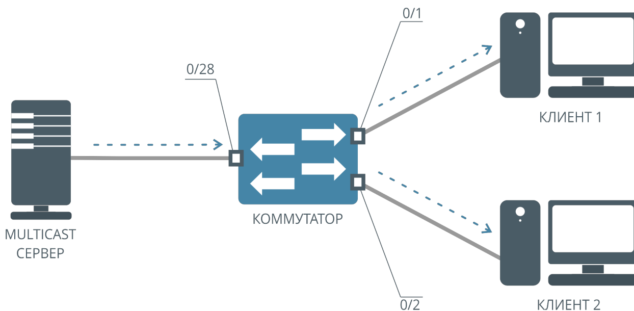
Рисунок 37. Схема передачи Multicast-трафика
