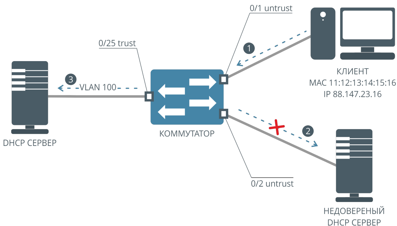
Рисунок 56. Схема работы DHCP Snooping
