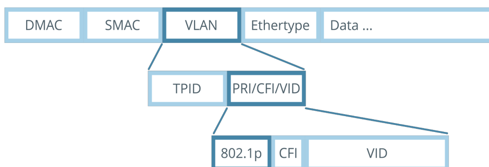
Рисунок 61. Положение метки 802.1p в теге 802.1q
