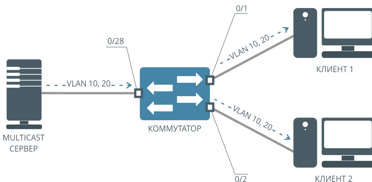
Рисунок 38. Схема подключения с двумя клиентами
