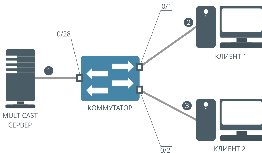
Рисунок 42. Схема работы профилей IGMP
