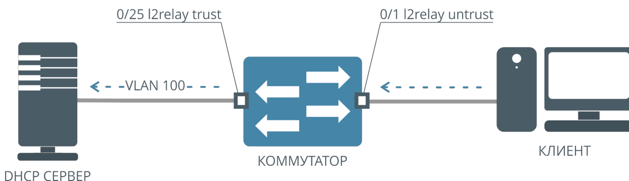
Рисунок 57. Схема работы DHCP L2 Relay
