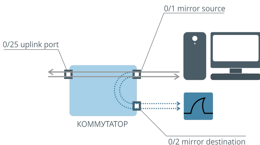
Рисунок 15. Механизм зеркалирования
