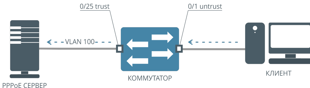
Рисунок 54. Упрощенная схема для иллюстрации работы PPPoE IA
