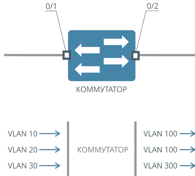
Рисунок 27. Схема работы выходной трансляции
