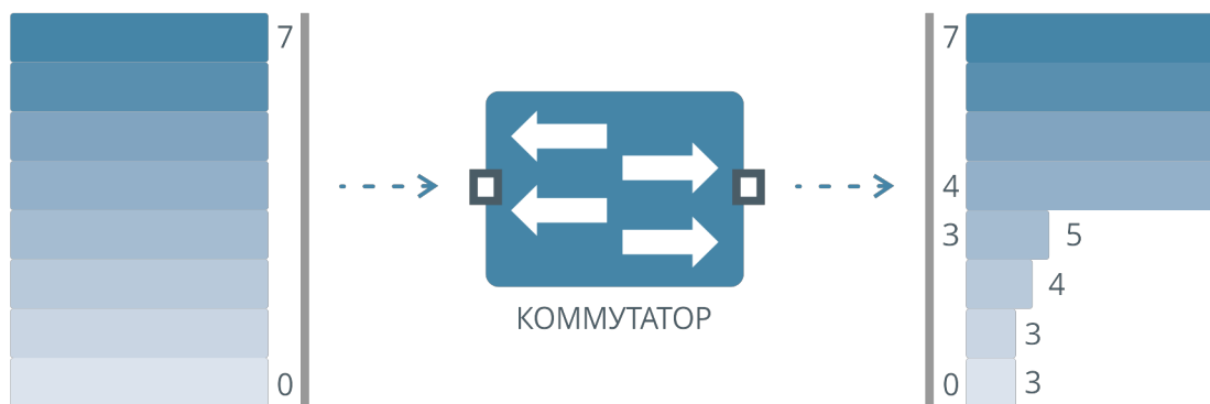
Рисунок 64. Алгоритмы Strict Priority и Weighted Round Robin одновременно
