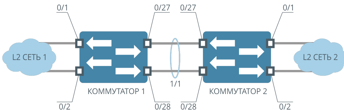
Рисунок 14. Пример статической агрегации каналов для двух L2-сетей
