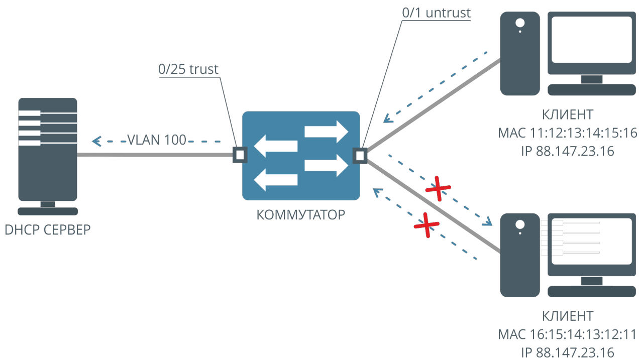
Рисунок 58. Схема работы DHCP IP Source Guard
