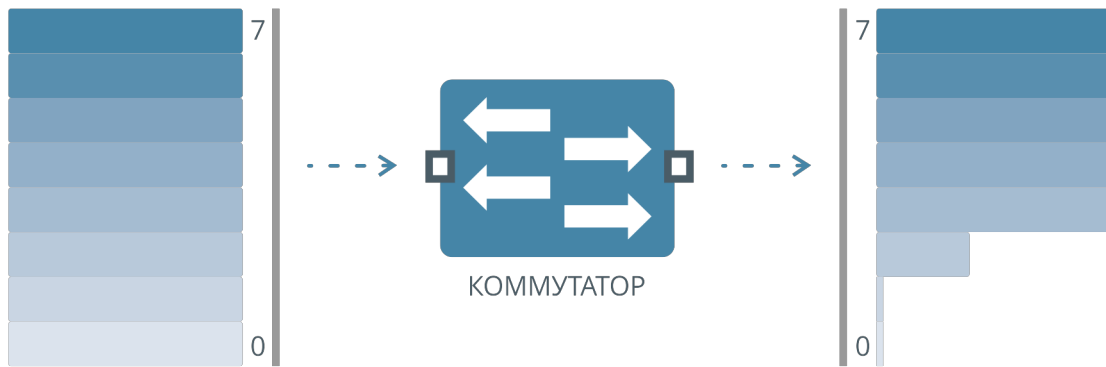
Рисунок 62. Алгоритм Strict Priority
