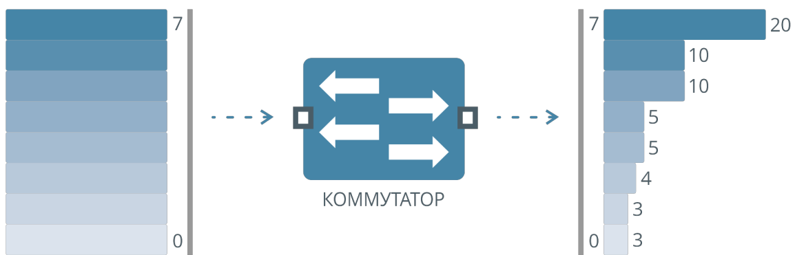
Рисунок 63. Алгоритм Weighted Round Robin
