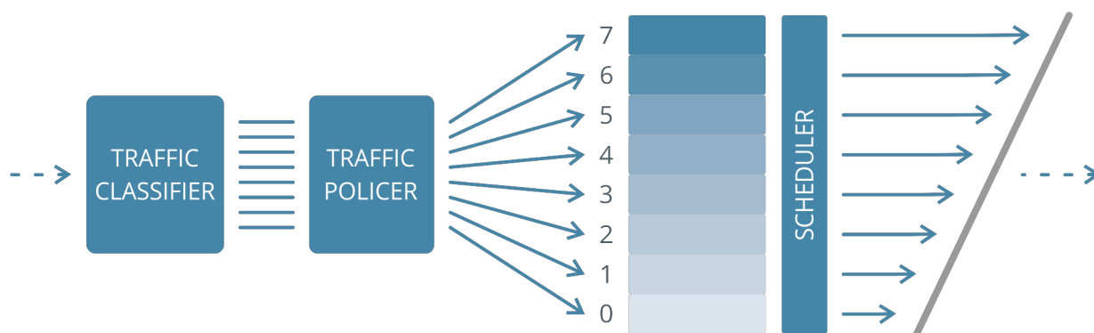
Рисунок 61. Механизм работы QoS на коммутаторах АЛСиТЕК
